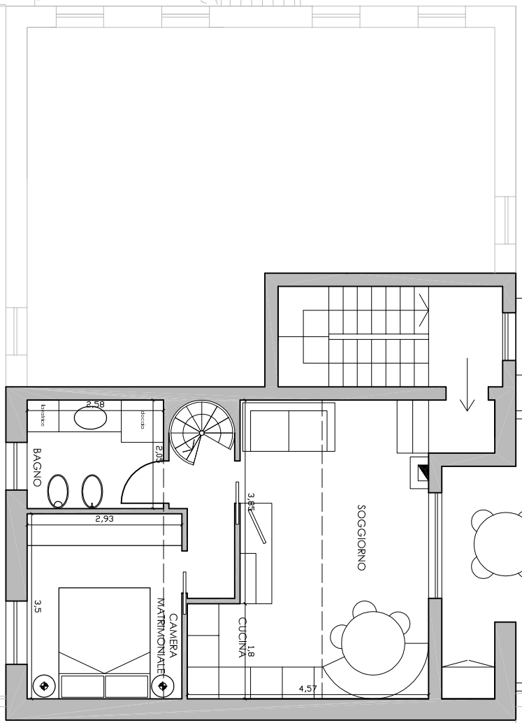
"La Filanda" PIANTA APPARTAMENTO "O4" PIANO PRIMO 1:100
