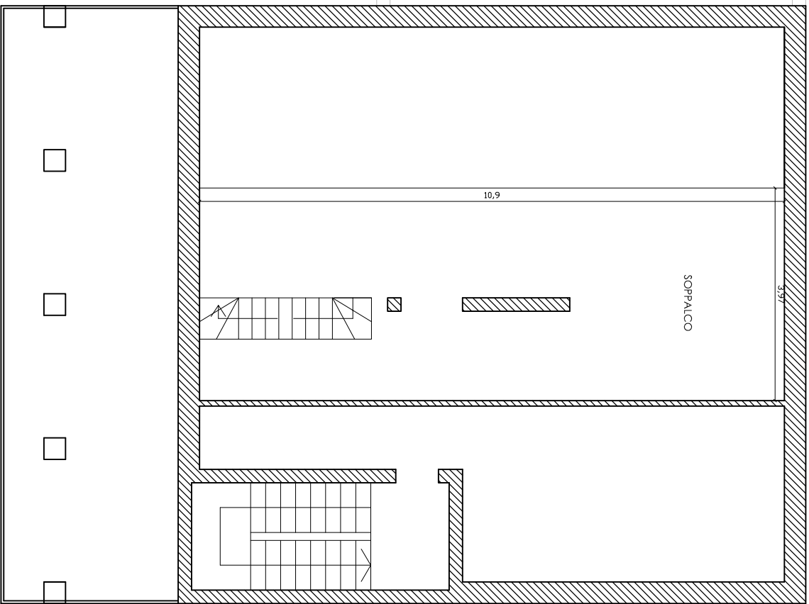
PIANTA APPARTAMENTO "NB" PIANO PRIMO SOPPALCATO 1:100
