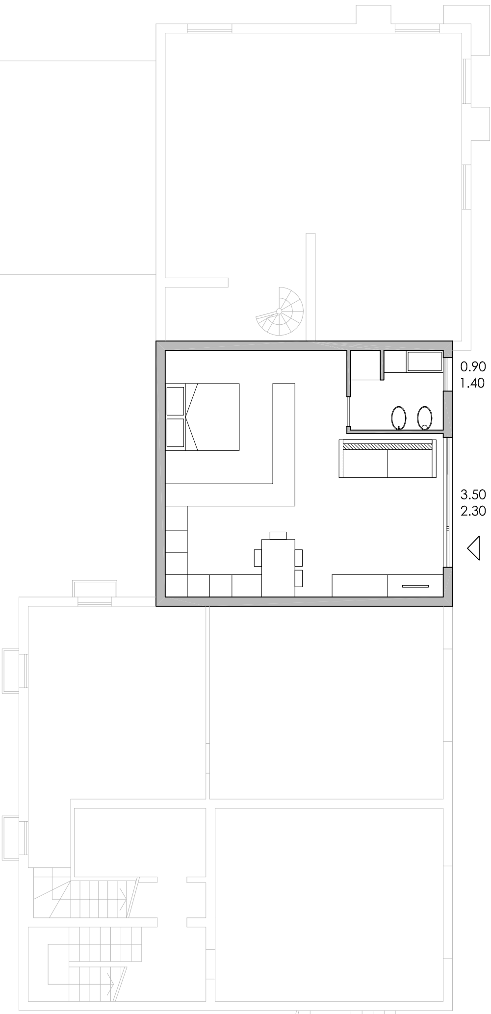
PIANTA MONOLOCALE "3" PIANO SEMINTERRATO 1:100
